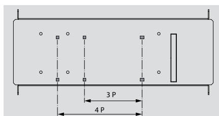
Fixation dans le 2 ème trou
