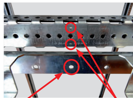
Trou représentant le milieu de l'équerre
